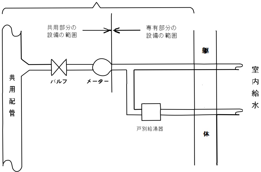
別図第1 給水管等の分界（別表第2（専有部分の専用に供される設備の帰属）第一号関係） 戸別メーターボックス内
