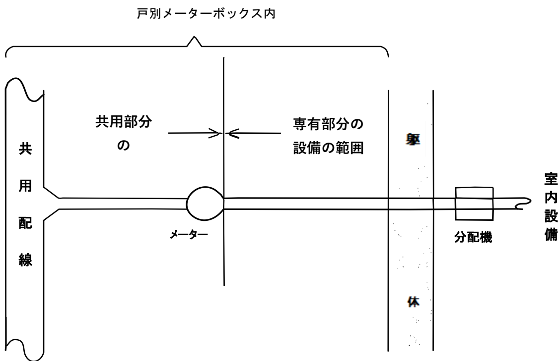
別図第4 電気設備の分界（別表第2（専有部分の専用に供される設備の帰属）第六号関係）
